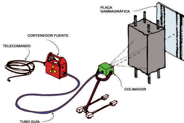
Fig. 1. Esquema de un equipo de gammagrafado de hormigón. La fuente cuando no se usa está alojada en el contenedor y al realizarse la medición ésta es desplazada al colimador mediante un telecomando y un tubo guía.
