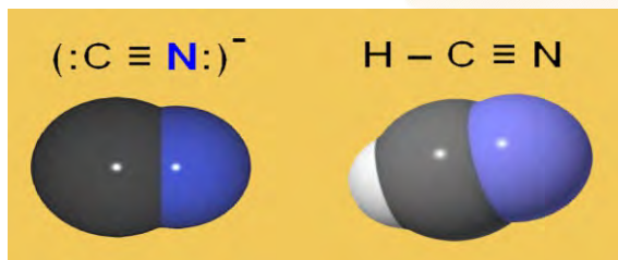
Fig. 1 Ion cianuro y cianuro de hidrógeno
