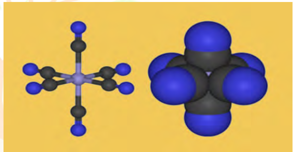
Fig. 2 Dos representaciones del ion ferrocianuro
