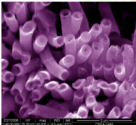
Fig. 3 - Micrografía electrónica de nanotubos de SnO 2 . Magnificación 40.000x
