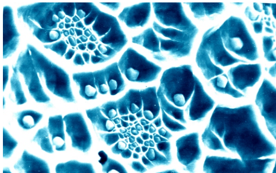
Fig. 2 - Micrografía electrónica de la superficie de fractura dúctil de un acero estructural. Se observan las cavidades características (dimples) de este modo de rotura.
