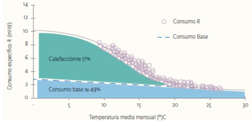
Figura 23 Variación de los consumos específicos R (marcados en la figura con círculos colorados). La línea de trazos cortos es una extrapolación del consumo base y muestra su dependencia con la temperatura. Los consumos específicos que se grafican son los promedios diarios mensuales como función de la temperatura media mensual. 1 El área sombreada indica el consumo asociado con la calefacción. Los datos corresponden a todo el país, exceptuado la zona sur del país. 1
