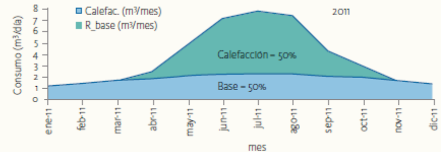
Figura 24 Consumos específicos diarios R+C+EO a lo largo de 2011. Los consumos de los meses de verano permiten caracterizar los consumos base. Si se atribuyen los consumos adicionales en los meses más fríos al uso de la calefacción, se observa que el consumo de calefacción de edificios varía entre 48% y 60% del total del consumo R+C+EO, dependiendo de la rigurosidad del invierno de cada año. Los datos corresponden a todo el país. 1
